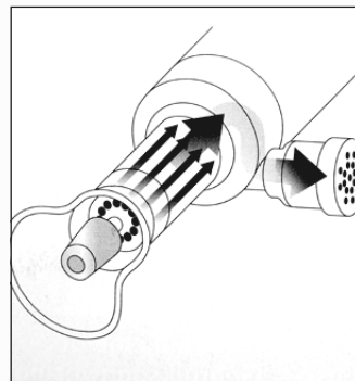
Das Funktionsprinzip einer Turbine, in der Zeichnung einmal sichtbar gemacht.
